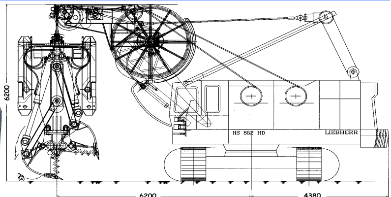
Montage sur grue Liebherr 855 Liebherr 855 crane assembling
